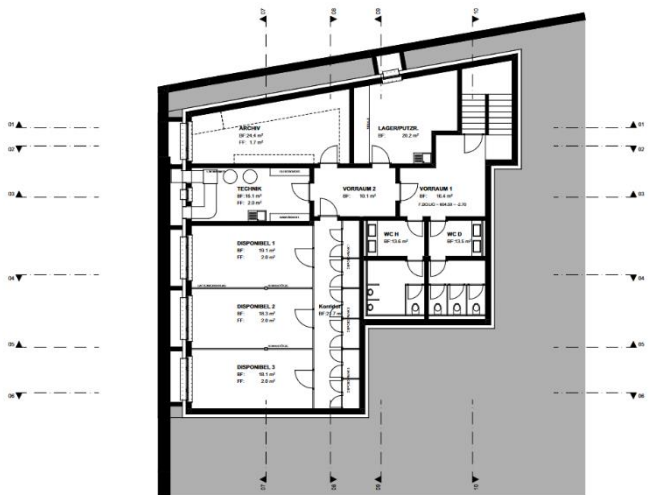
Ansicht Untergeschoss
