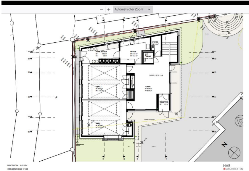
Ansicht Erdgeschoss
